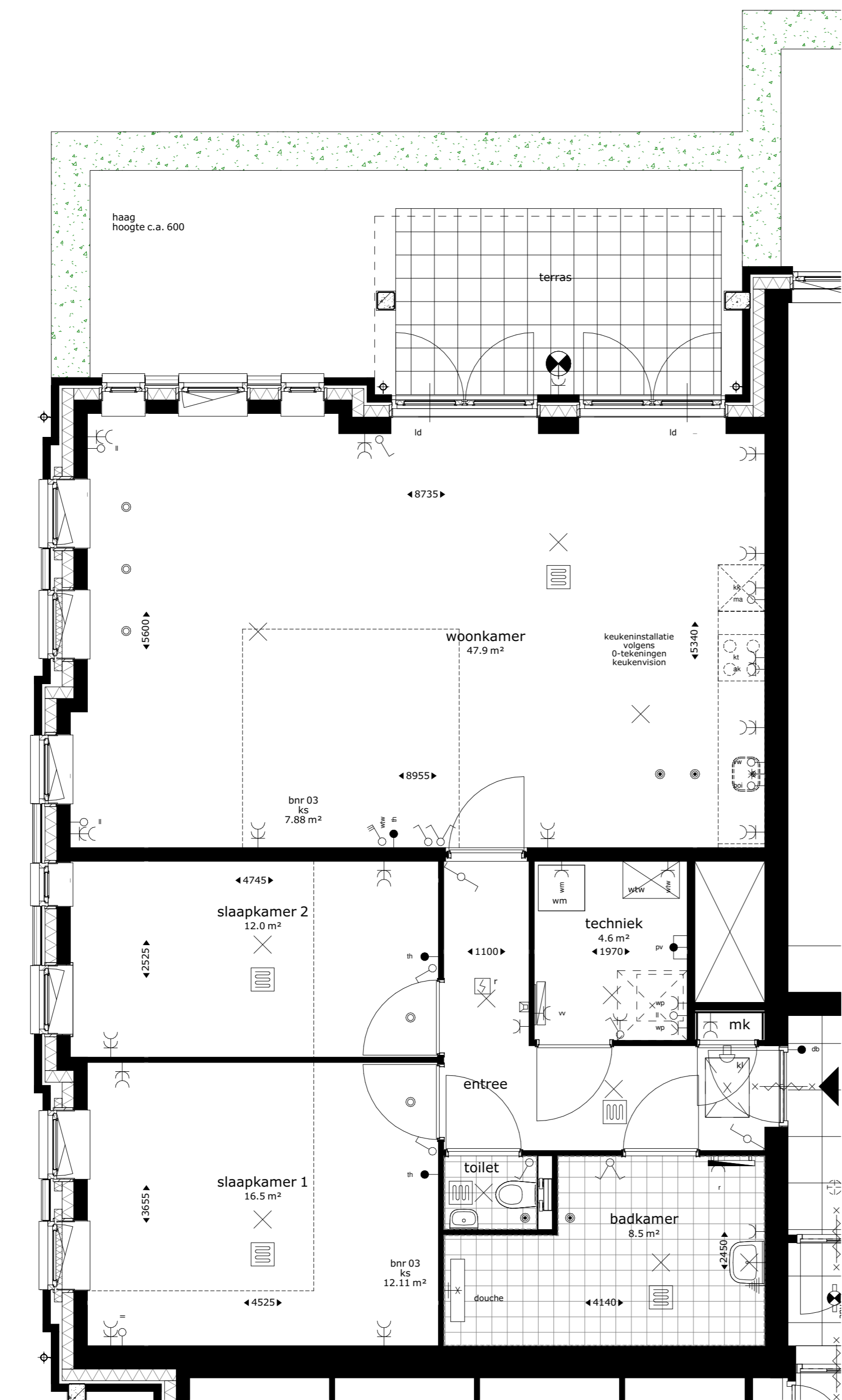
bouwnr 03 1 : 50
